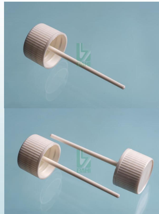
Código: 41.5018.4BC Medida: Ø | 18MM - H13.6MM
